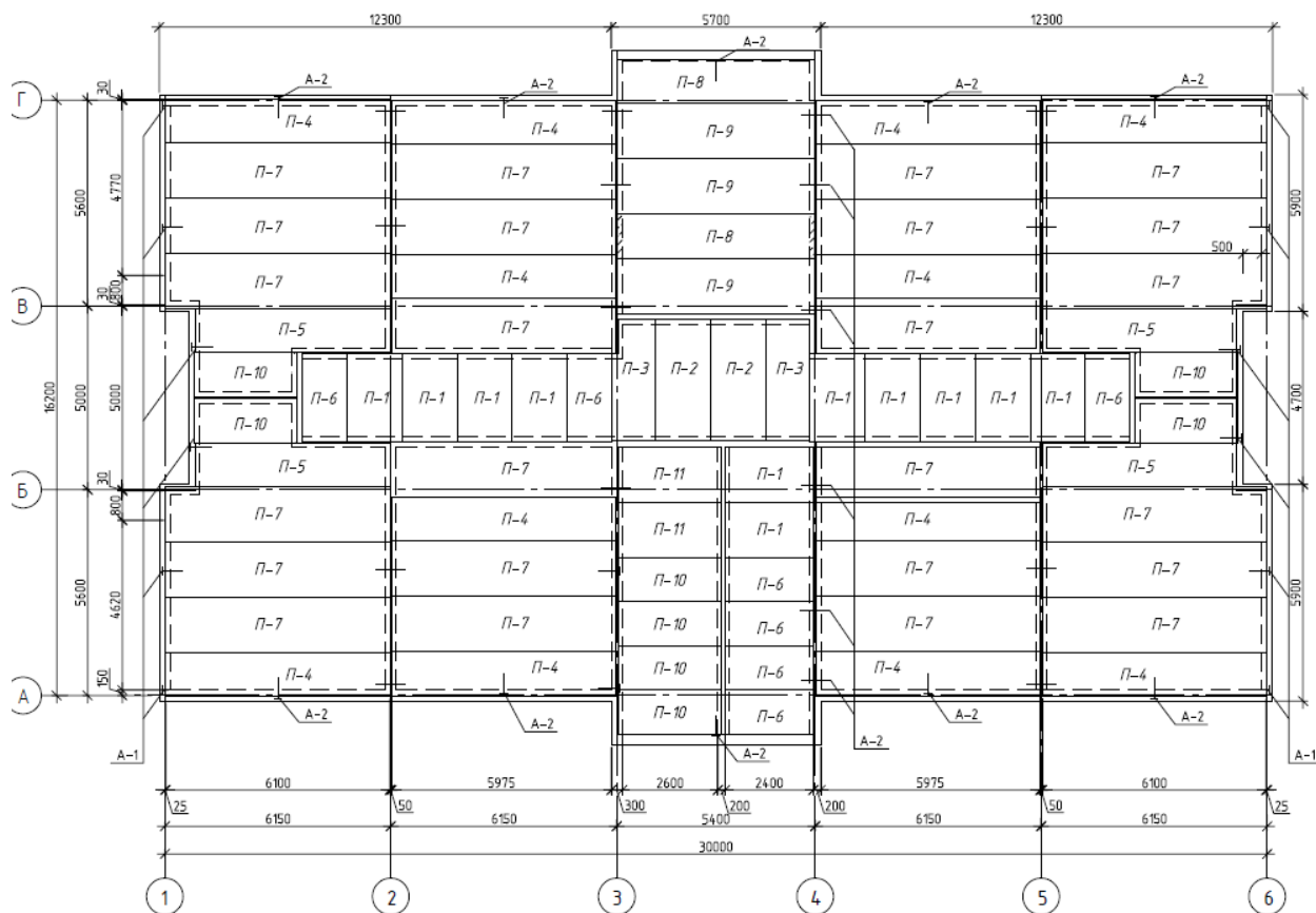
Рис.8 Схема расположения плит перекрытия на отм.0.000. Обследование межэтажного перекрытия
