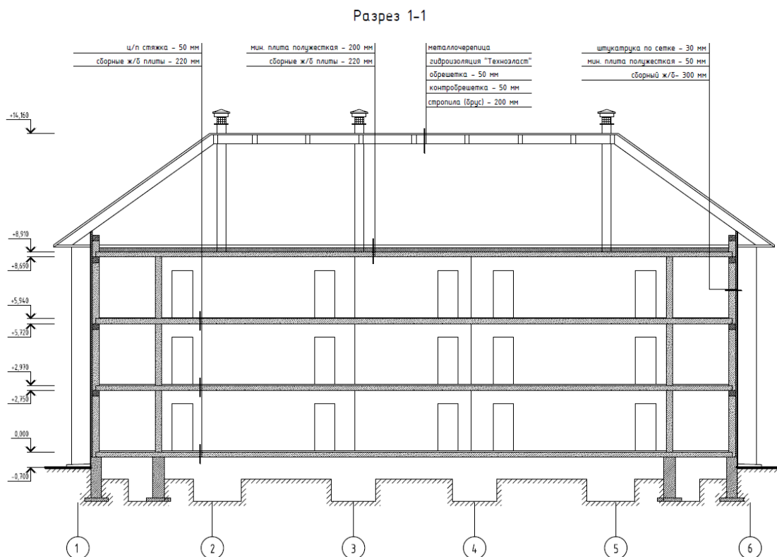
Рис.4 Разрез 1-1
