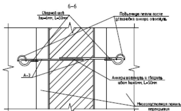
Рис.10 Узел анкеровки плит перекрытия. Обследование межэтажного перекрытия
