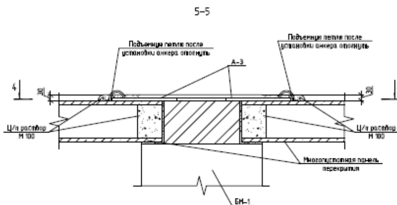
Рис.9 Узел анкерки плит перекрытия. Обследование межэтажного перекрытия
